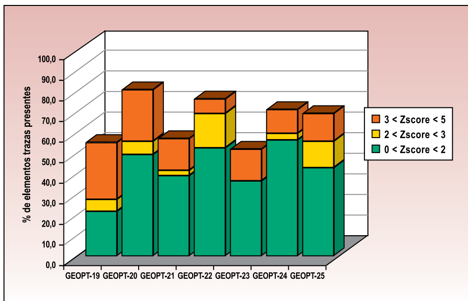
Figura 44 Gráficas de comparación de porcentajes de valores Z-Score en el estudio de intercomparación organizado por la "International Association of Geonalysts" (2006-2009): a) Elementos mayoritarios, b) elementos traza.
